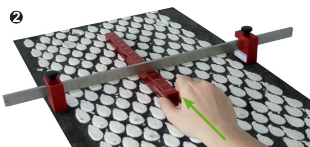
Direction of movement of the wedge / Schieberichtung des Keils
